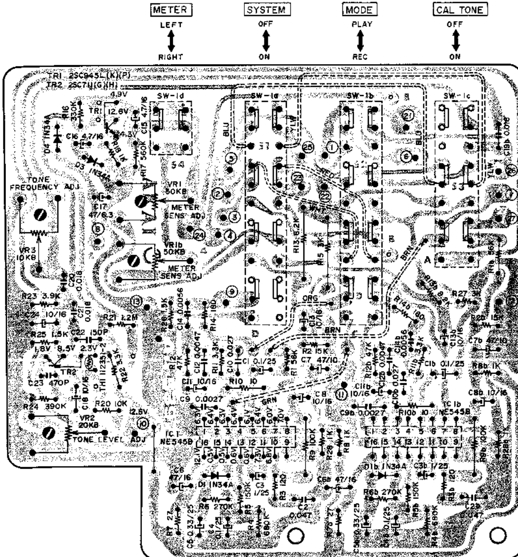
7) DOLBY N.R. P.C BOARD AA-5397
