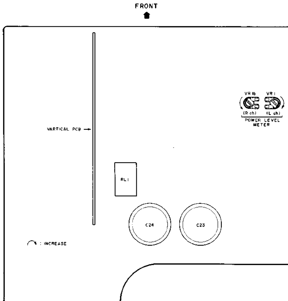
Fig. 6-2 Main-Amp PCB
