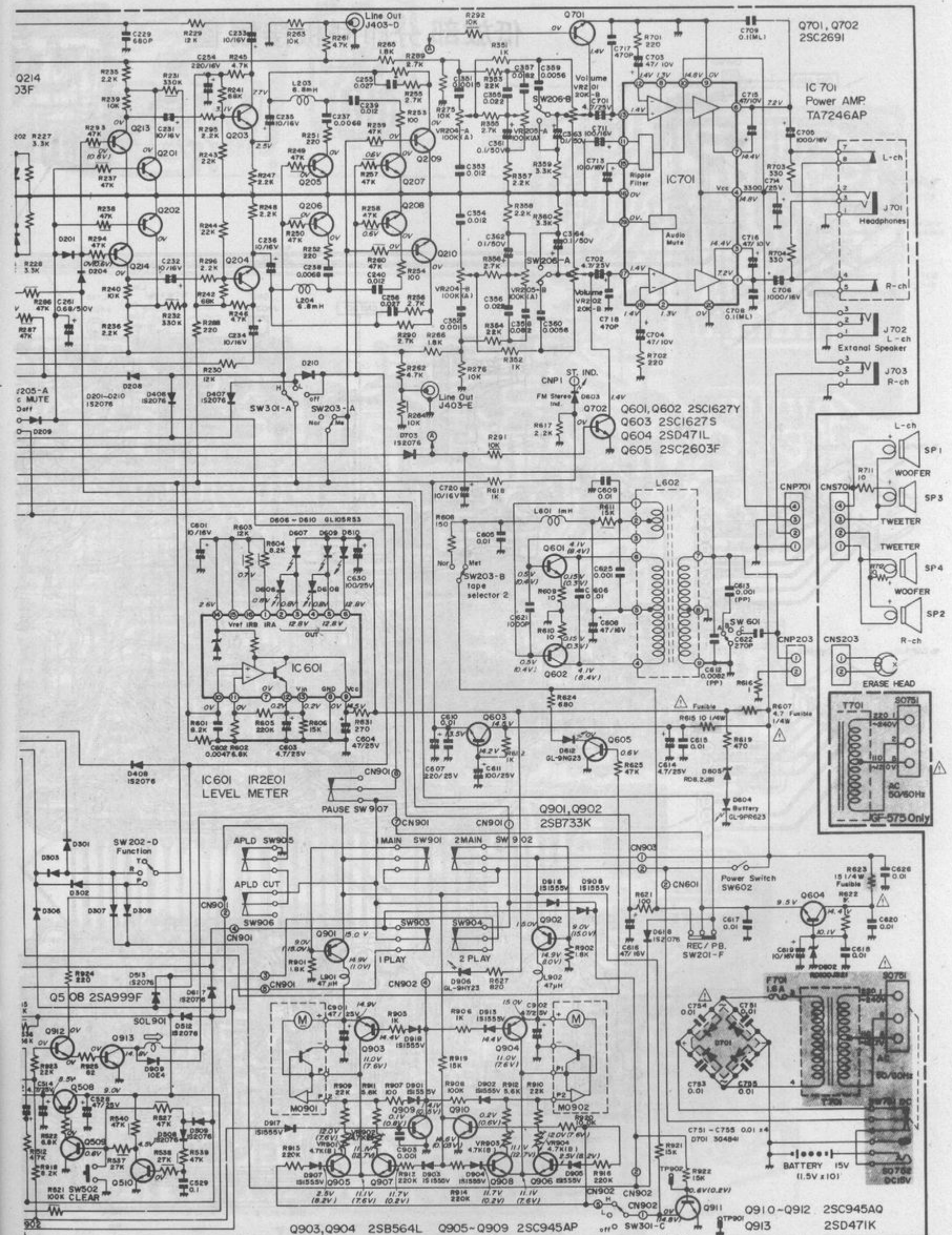
低放部分电原理图
