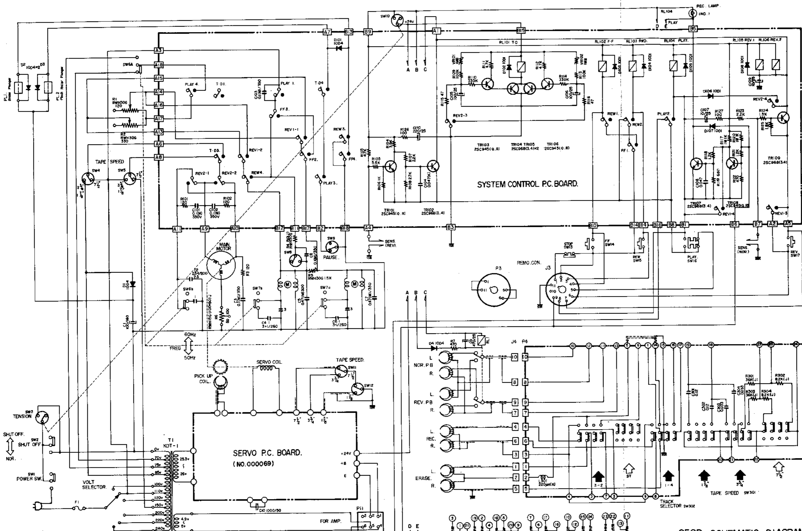
250D SCHEMATIC DIAGRAM (MECHA. BLOCK DIAGRAM.) No. 2-1 14020380
