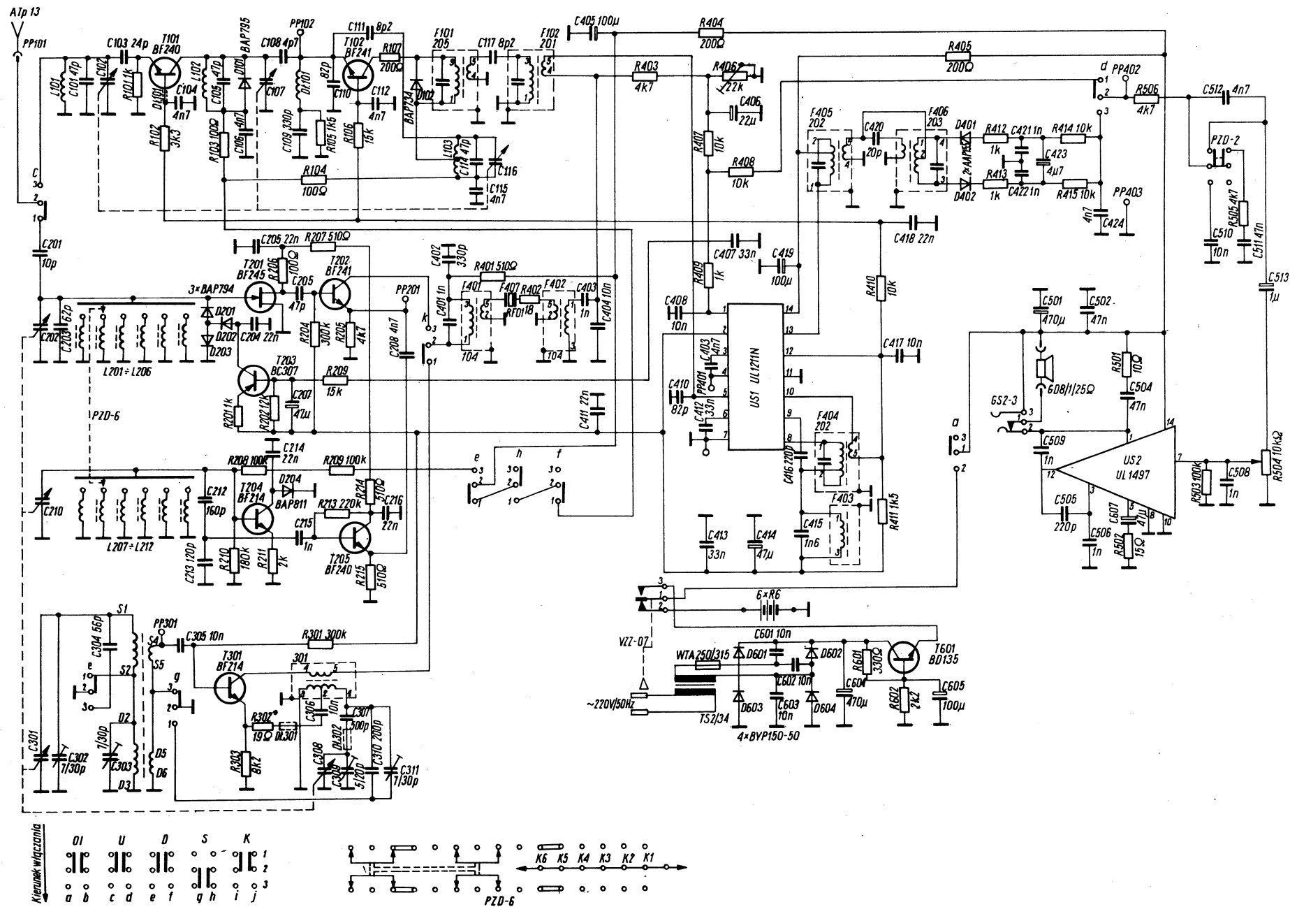
Schemat odbiornika radiofonicznego Roksana R-601
