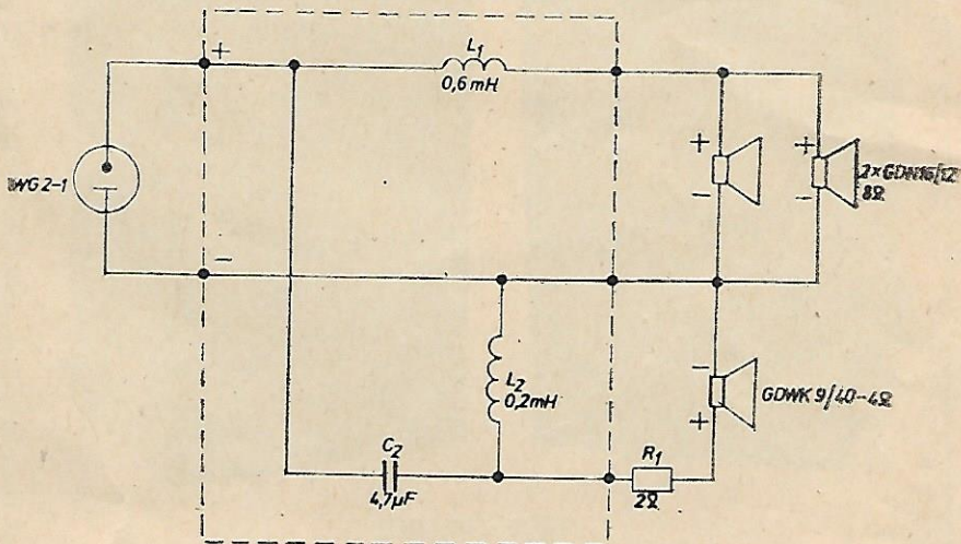
Schemat ideowy ZG25-C
