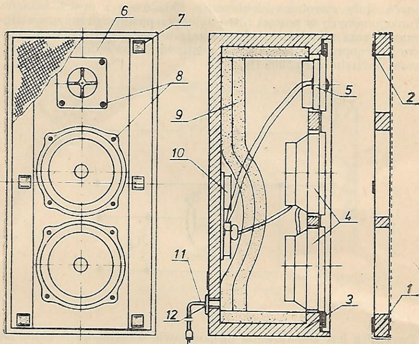
Rys. 4. Zestaw głośnikowy ZG25-C
