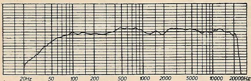
Rys. 3. Przykładowa charakterystyka elektroakustyczna zestawu głośnikowego ZG25-C
