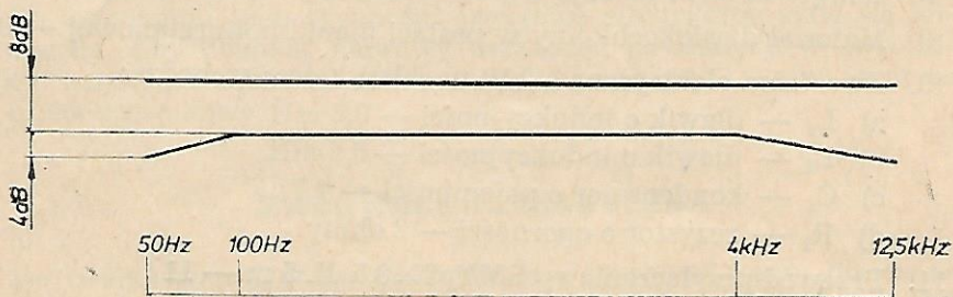
Rys. 2. Pole tolerancji
